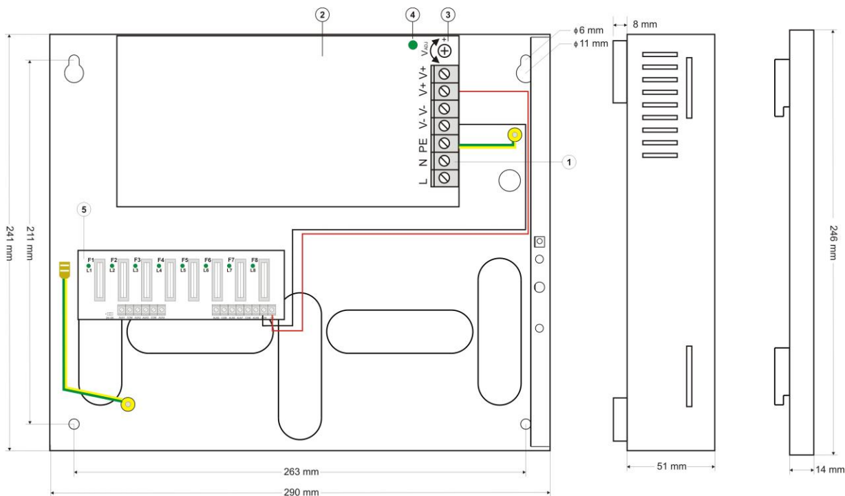
Bild 3. Netzteil-Ansicht
